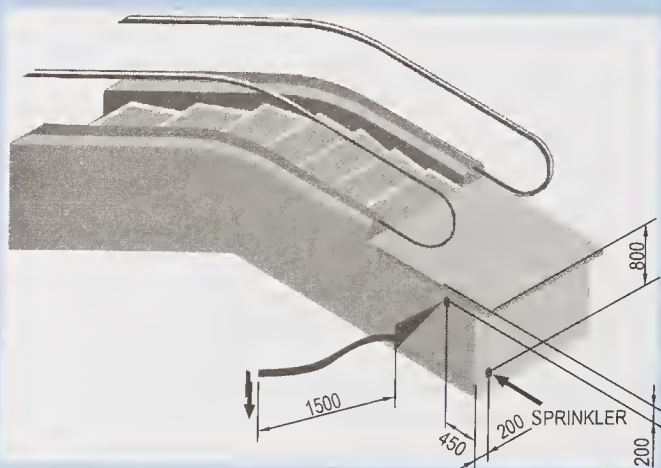
FIG. 13 SPRINKLER PIPING
